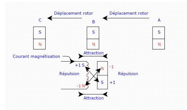
FIGURE 2. Séquence de déplacement du rotor (positions A, B, C) face à l'électro-aimant à noyau néodyme dont le champ propre est annulé par superposition. Le schéma reprend la même convention de polarité et d'interaction croisée que la Figure 1.
