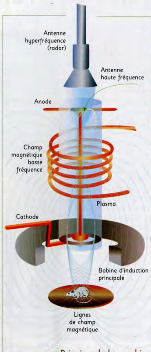
Principe de la machine
